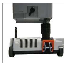
Rapido sganciamento della base dal corpo macchina
